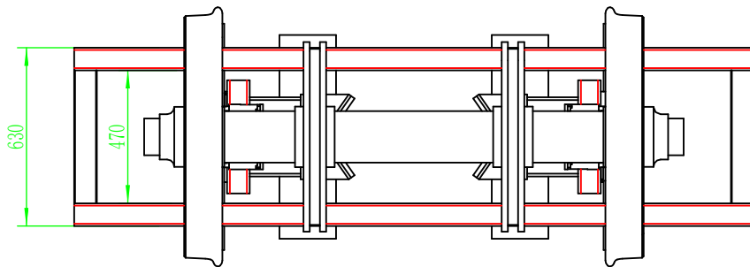
轮轴储运示意图
