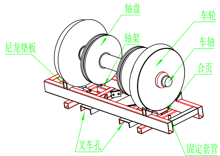
轮轴储运示意图
